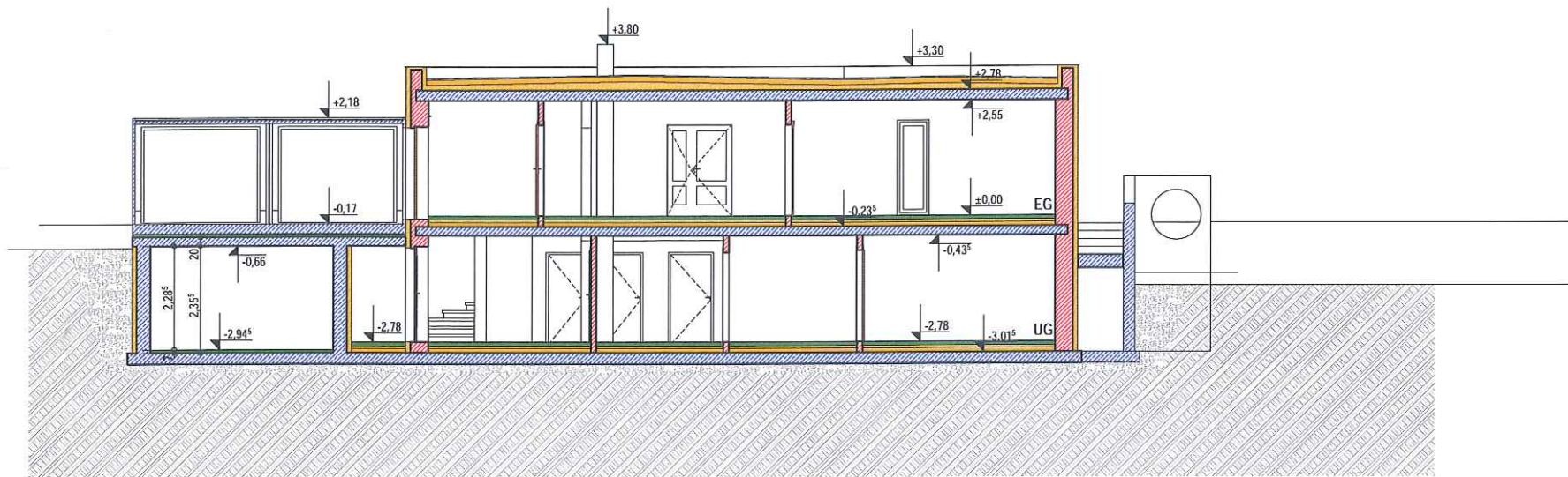
SCHNITT: A-A
