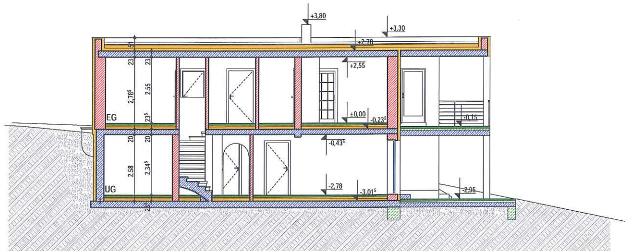
SCHNITT: B-B
