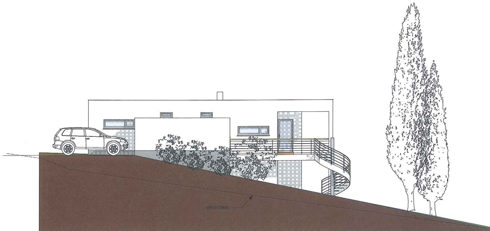
WESTANSICHT
